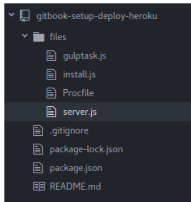
Figura 3.7: Estructura de directorios del plugin de Heroku.
