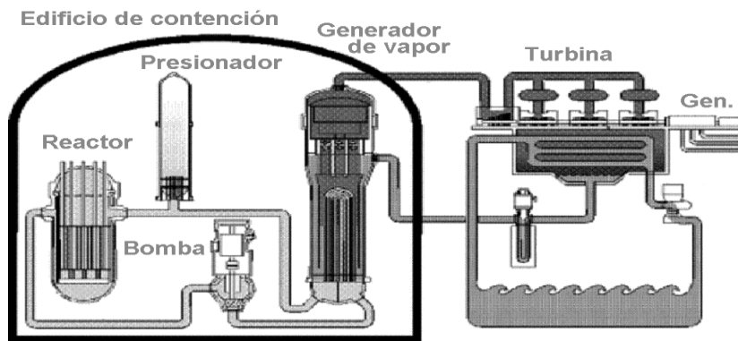
Ilustración 8. Motor nuclear. (21)
