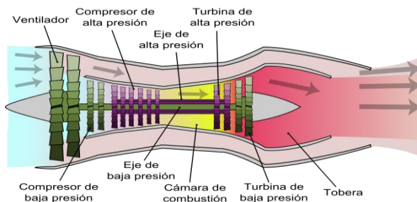
Ilustración 7. Turbina de gas. (22)
