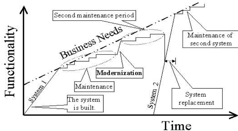
Figura 1: Ciclo de vida del sistema de software [13]
