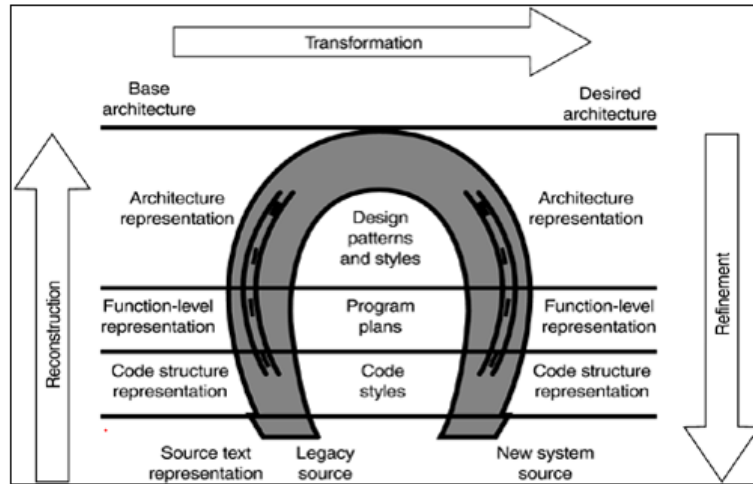
Figura 3: Modelo en herradura o HorseShoe Model [26]
