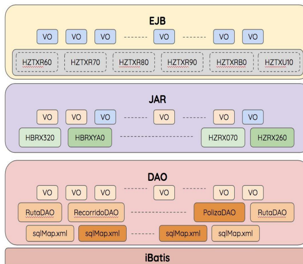
Figura 14 : Artefactos en plataforma DELTA/SIC
