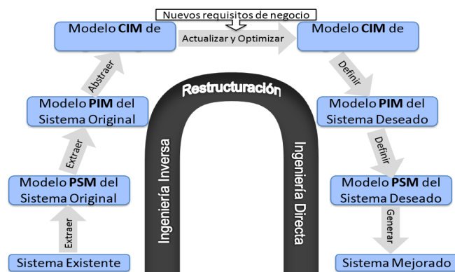
Figura 5: Modelo de Modernización en Herradura de ADM [31]
