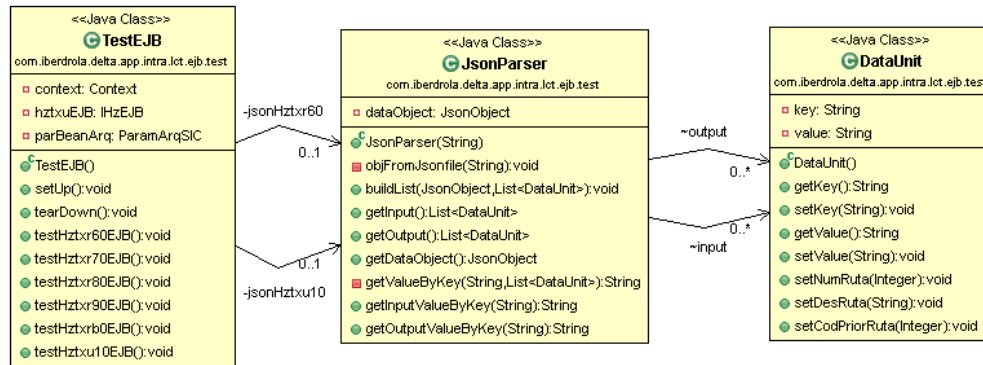
Figura 15: Interfaz JSON Parcer
