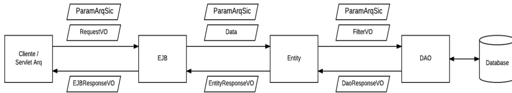
Figura 12: interacción de los componentes de la arquitectura
