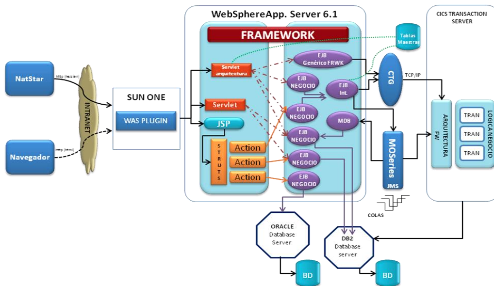
Figura 11: Arquitectura de destino de aplicaciones
