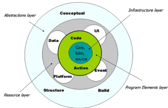
Figura 6: Arquitectura KDM 17
