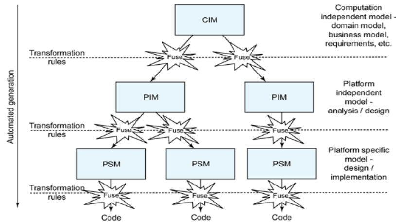
Figura 2 : Modelos MDA según nivel de abstracción 15
