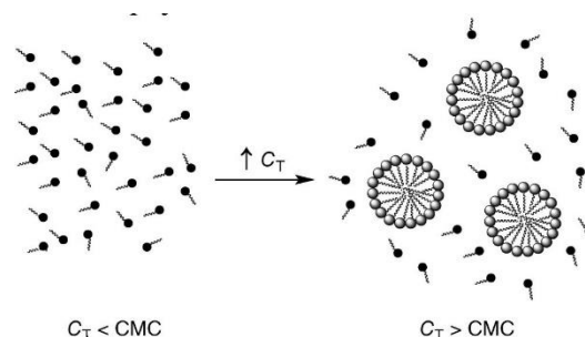
Fig. 8. - Representación del comportamiento del tensoactivo en disolución acuosa cuando se encuentra en forma iónica (izquierda) y cuando se forman las micelas (derecha) [4]. El comportamiento químico del SDS en disolución acuosa, es el de disociarse en aniones de dodecilsulfato ( \text{SD}^- ) y cationes de sodio ( \text{Na}^+ ). Este grado de disociación se ha estimado midiendo su conductividad eléctrica en disolución, con el fin de calcular el punto de concentración micelar crítica CMC. Como hemos visto, nos indica el punto de concentración de surfactante al cuál, las moléculas de SDS, dejan de comportarse como iones independientes, para asociarse formando estructuras micelares.
