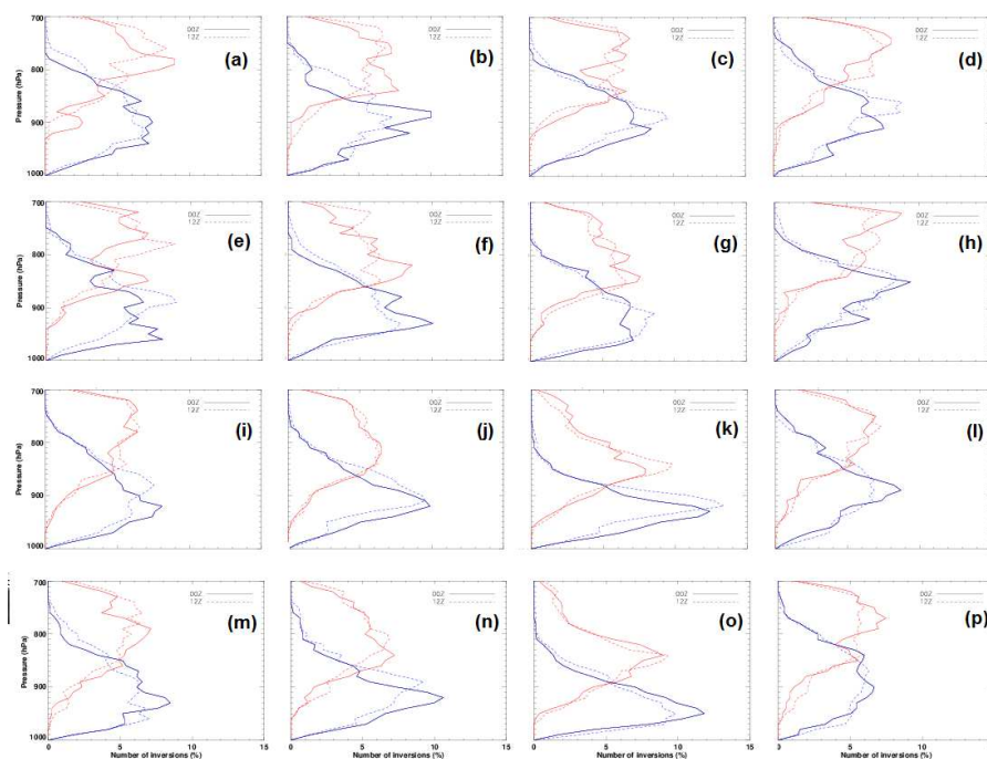
Fig. 3.8 Porcentaje de inversiones por niveles de presión, divididos en cuatro intervalos: ene-feb-mar (a, e, i, m), abr-may-jun (b, f, j, n), jul-ago-sep (c, g, k, o) y oct-nov-dic (d, h, l, p), en Azores (a-d), Madeira (e-h) e Islas Canarias: Santa Cruz (i-l) and Güimar (m-p). (ROJO) Inversión MBL, (AZUL) Inversión de Subsidencia. (Línea continúa) Sondeos nocturnos, (Línea discontinua) Sondeos diurnos.
