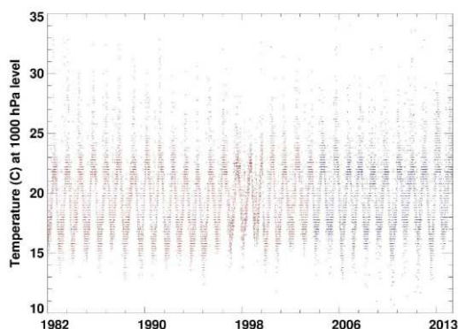
Fig. 2.4 Evolución de la temperatura, durante el período utilizado para caracterizar las inversiones MBL y TWI, a 1000 hPa. Se refleja el cambio de ubicación de la estación de Islas Canarias desde Santa Cruz a Güimar, en el año 2002.
