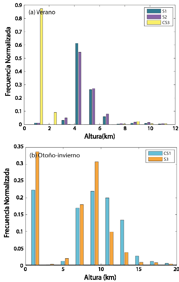
Fig. 3.13. (Barreto et al., 2017) Histogramas normalizados de frecuencia de nubes identificadas, en la columna vertical, en los escenarios de (a) verano y (b) otoño-invierno, bajo condiciones limpias y de polvo, entre 2007 y 2014.
