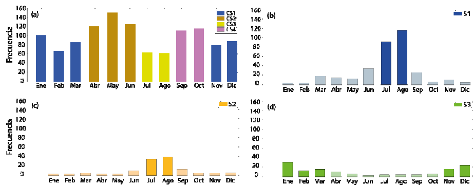
Fig. 3.9. (Barreto et al., 2017) Histogramas de frecuencia absoluta, para cada escenario definido de acuerdo con los datos de AERONET, de 2007 a 2014.
