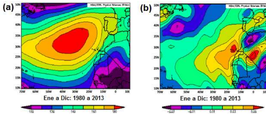
Fig. 2.2 Situaciones sinópticas de la región de estudio, con datos de reanálisis. (a) Altura geopotencial (m) correspondiente a la superficie isobárica de 1000 hPa. (b) Subsistencia en Pa/s.
