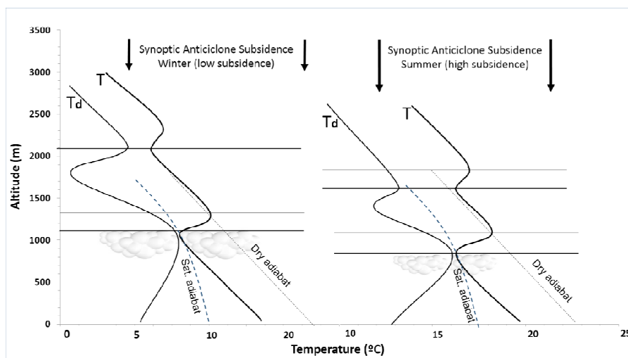
Fig. 3.6. Sección vertical esquemática que representa dos perspectivas de la primera y segunda capa de inversión, con baja (izda) y alta (dcha) subsidencia. Una subsidencia elevada presiona la masa de aire situada por debajo. La cima de la primera inversión, un nivel seco, desciende a lo largo de la adiábata seca, sin embargo, la base, que está en un nivel muy húmedo, desciende a lo largo de la adiábata saturada. Este calentamiento diferencial produce un reforzamiento de esta capa de inversión.
