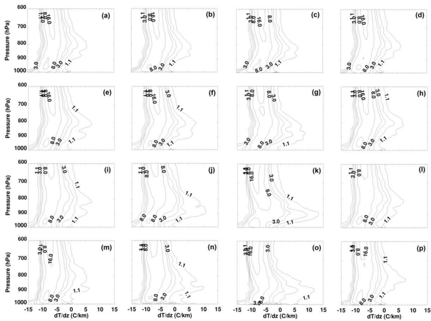
Fig. 3.2 Diagrama de contorno de frecuencia por altitud (diagrama CFA) de la estabilidad ( dt/dz^{-1} ), dividida en cuatro intervalos: ene-feb-mar (a, e, i, m), abr-may-jun (b, f, j, n), jul-ago-sep (c, g, k, o) y oct-nov-dic (d, h, l, p), en Azores (a-d), Madeira (e-h) e Islas Canarias: Santa Cruz (i-l) y Güimar (m-p). Las isolíneas representan la frecuencia (%) de las observaciones, a un nivel determinado, en las que se detectan estabilidades en intervalos de 1 \text{ K km}^{-1} .
