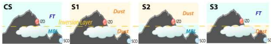
Fig. 2.6. Cuatro escenarios definidos en Tenerife (Islas Canarias) para estudiar la influencia de las intrusiones de polvo mineral procedente del Sáhara en la estructura térmica vertical. Se sombreen en azul las condiciones limpias; en la capa límite marina (SCO: Santa Cruz) y en la Troposfera libre subtropical (IZO: Izaña). Las condiciones polvorientas son sombreadas en naranja. El escenario CS muestra condiciones limpias en la MBL y troposfera libre. Los tres escenarios restantes: S1, S2 y S3 están afectados por el polvo sahariano.
