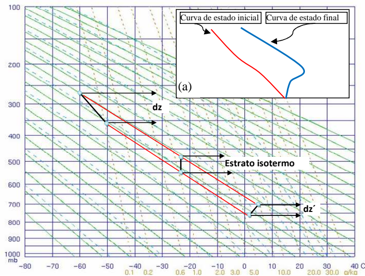
Fig. 1.5 Calentamiento adiabático diferencial de un estrato. (a) Modificación del perfil vertical de temperatura.
