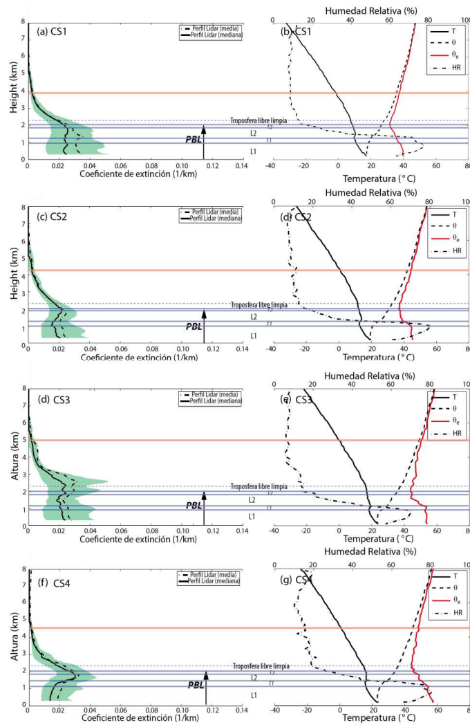
Fig. 3.10. (Barreto et al., 2017). Perfiles de extinción y perfiles verticales de temperatura ( T ), temperatura potencial ( \theta ), Temperatura potencial equivalente ( \theta_e ) y humedad relativa (HR) para cada escenario limpio. La línea punteada azul representa la altitud de la estación IZO. Las líneas horizontales azules representan diferentes capas y la línea horizontal roja indica el nivel promedio de 0^\circ\text{C} , extraídas de los sondeos verticales. El área verde sombreada está delimitada por los valores del percentil 20^\circ y 80^\circ de la extinción total lidar en cada nivel.
