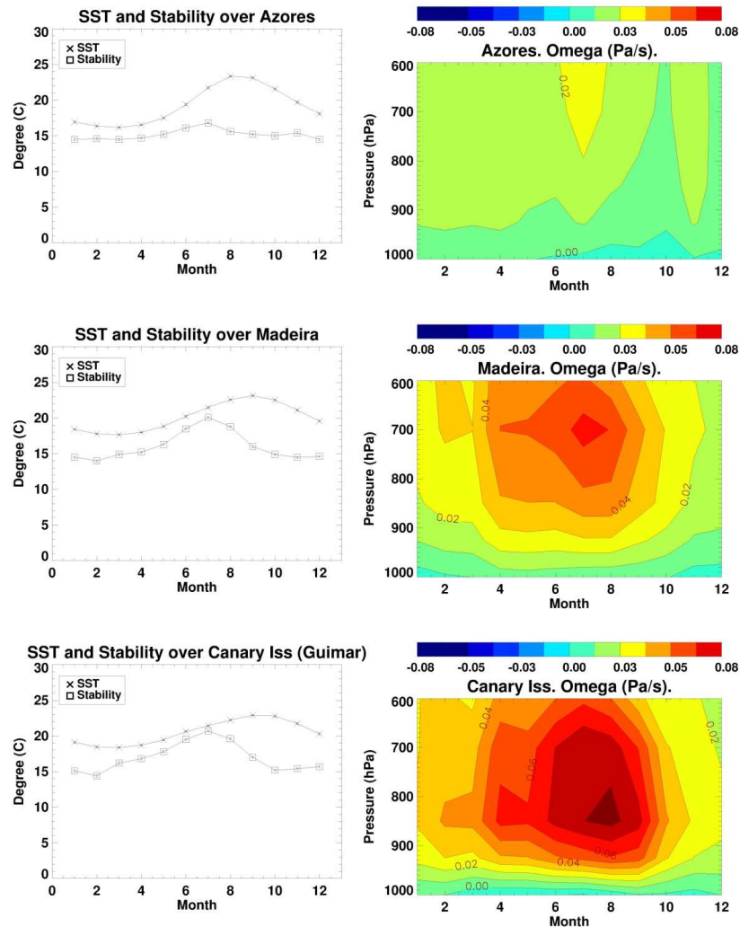
Fig. 3.4. (Izquierda) Variación anual de la SST ( ^{\circ}\text{C} ) y la estabilidad ( ^{\circ}\text{C} ). Los datos fueron promediados en Canarias, para calcular el parámetro SST, desde 27.6 a 29.5^{\circ}\text{N} y 13.1 a 16.9^{\circ}\text{E} , en Madeira desde 29.5 a 35.2^{\circ}\text{N} y 15 a 16.9^{\circ}\text{E} y, en Azores, desde 35.2 a 41.0^{\circ}\text{N} y 22.5 hasta 30.0^{\circ}\text{E} . Las barras de error representan el error estándar. (Derecha) Ciclo anual de la velocidad vertical ( \text{Pa s}^{-1} ) calculado con la base de datos de reanálisis del NCEP. En reanálisis, los valores para las Islas Canarias han sido tomados entre 27.5 a 30.0^{\circ}\text{N} y 12.5 a 17.5^{\circ}\text{E} , en Madeira desde 30.0 a 35.0^{\circ}\text{N} y 15 a 17.5^{\circ}\text{E} y, en Azores, desde 35.0 a 40.0^{\circ}\text{N} y 22.5 a 30^{\circ}\text{E} ; datos promediados por estación en el rango temporal analizado en este estudio (Tabla 2.1).
