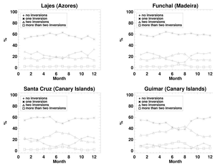
Fig. 3.1 Variación estacional de los porcentajes de sondeos con cero, una, dos o más de dos capas de inversión, en el rango de presiones entre 1000 y 700 hPa, en Islas Canarias (dos localizaciones), Madeira y Azores.
