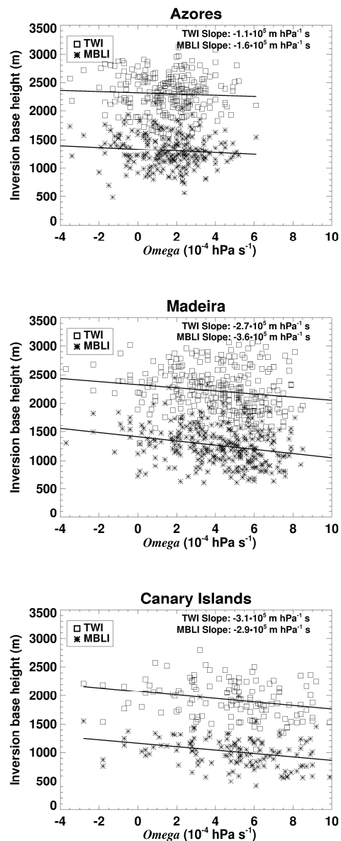
Fig. 3.7. Altura de la base de la inversión MBL (MBLI) (*) y TWI (□) vs velocidad vertical (omega) (hPa s -1 ) hasta el nivel de 700 hPa, en Azores, Madeira e Islas Canarias (Güimar).
