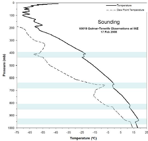
Fig. 1.3 Perfil de temperatura y temperatura del punto de rocío en la estación de Tenerife, a las 0000 UTC, el 17 de febrero de 2008.
