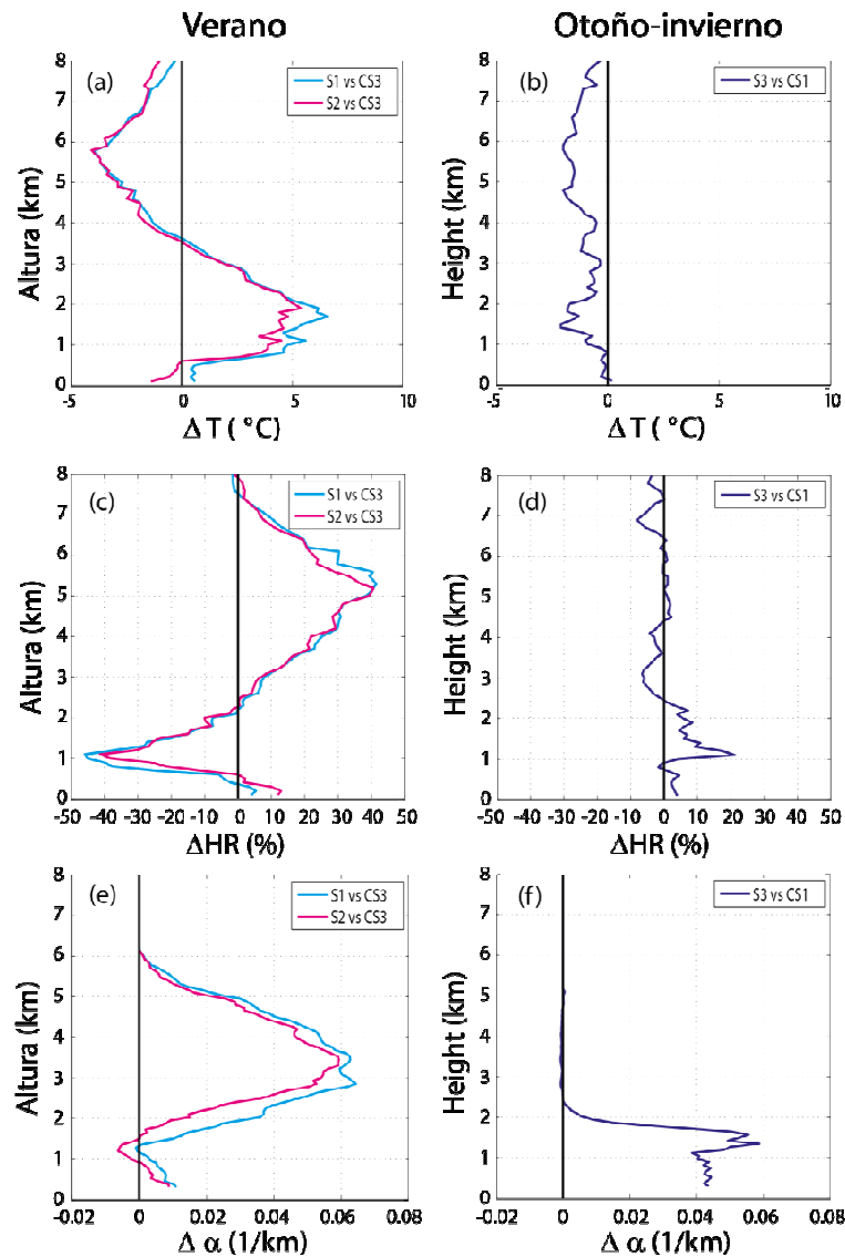
FIG. 3.12. (Barreto et al., 2017) Diferencias absolutas entre escenarios de polvo y limpios de los parámetros temperatura (a y b), humedad relativa (c y d) y coeficiente de extinción (e y f) para verano (1ª columna) y otoño-invierno (2ª columna), respectivamente.
