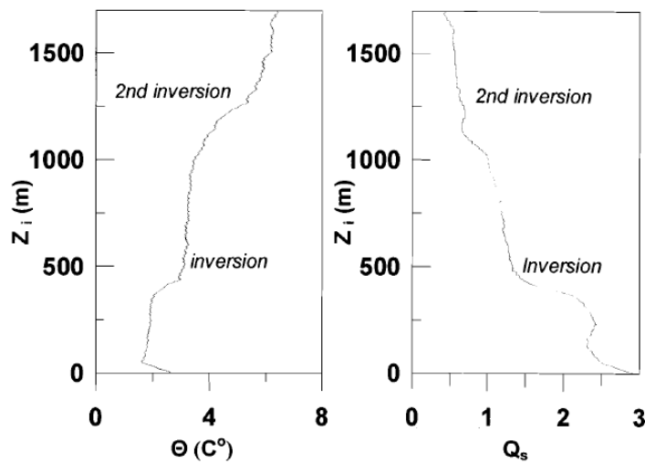
Fig. 1.6 (Arriba) Diagrama de contorno de frecuencia por altura de la estabilidad en Kapinga (Micronesia), procesado usando diferencias centradas cada 20 hPa en 475 sondeos. (Adaptado de Johnson et al., 1995). (Abajo) Ejemplo de una situación clásica en Anholt (Dinamarca) mostrando la detección de la altitud de las inversiones, en perfiles de radiosondeo. Temperatura potencial (izda) y humedad específica (drcha) (Tomado de Sempreviva y Gryning, 2000).
