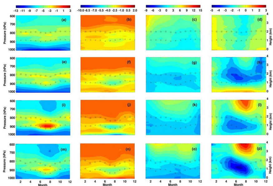
Fig.3.3 Ciclo anual del gradiente de temperatura ( \text{K km}^{-1} ), primera columna; gradiente de la razón de mezcla dr dz^{-1} ( \text{g kg}^{-1} \text{km}^{-1} ), segunda columna; y componentes del viento zonal y meridional ( \text{m s}^{-1} ), tercera y cuarta columnas, respectivamente. Todas las figuras han sido calculadas usando solamente datos de sondeos con dos inversiones simultáneas identificadas en el rango entre 1000 y 700 hPa, en Azores (a–d), Madeira (e–h) e Islas Canarias: Santa Cruz (i–l) y Güimar (m–p). Las líneas de puntos indican la altitud promedio de la base de la primera (*) y segunda ( \square ) inversión. Las barras de error representan el error estándar.
