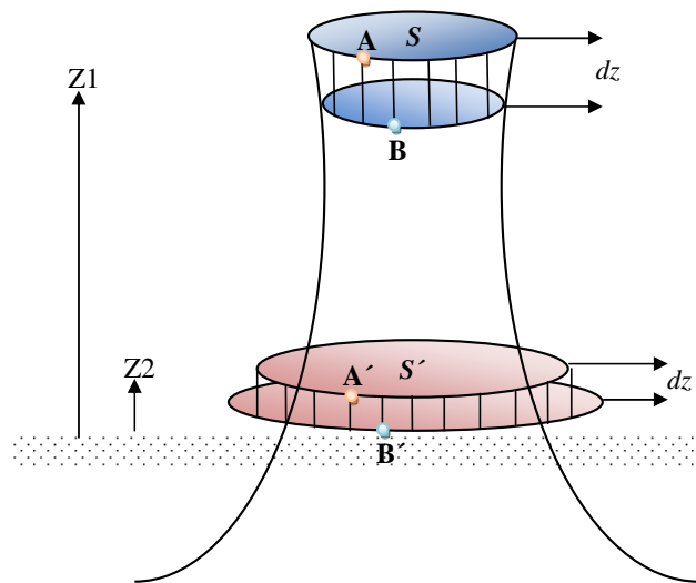
Fig. 1.4 Compresión adiabática de un estrato.
