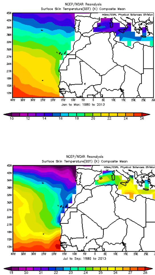
Fig.3.5. Composición de la media de la SST, desde 1980 hasta 2013, durante el invierno (panel superior) y durante el verano (panel inferior).
