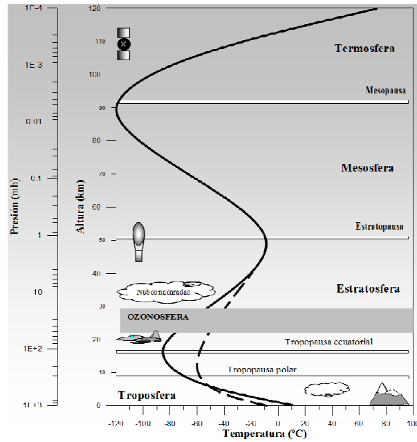
Fig 1.1 (Guerra et. al, 2002) Variación vertical típica de la temperatura atmosférica hasta 120 km de altura.
