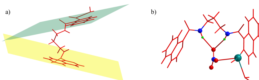
Figura 79. Compuesto 5b . a) Ángulo diedro generado entre los planos medios de los anillos de isoquinolina. b) Interacción de enlace hidrógeno \text{N-H}\cdots\text{O}_{(\text{nitrato})} , un átomo de oxígeno del contraion forma un enlace bifurcado con dos átomos de nitrógeno del grupo amida.
