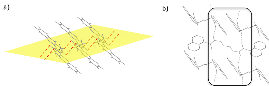
Figura 33. Representación de los motivos supramoleculares para enlaces de hidrógeno NH\cdots O (amida). a) Motivo en hojas \beta , los anillos aromáticos se alejan del plano definido por la porción cadena alifática-grupo amida (en amarillo). b) Motivo red 4,4, se observa que los anillos heterocíclicos se acomodan entre las cadenas alifáticas por la parte superior e inferior.
