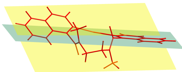
Figura 84. Compuesto 4g . Ángulo diedro generado entre los planos medios de los anillos de isoquinolina
