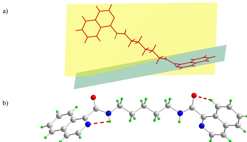
Figura 71. Compuesto 1d . a) Ángulo diedro generado entre los planos medios de los anillos de isoquinolina. b) Representación del enlace de hidrógeno intramolecular N-H (amida) ···N (isoquinolina)
