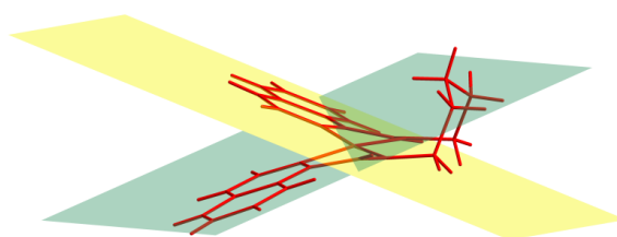
Figura 90. Compuesto 7d . Ángulo diedro generado entre los planos medios de los anillos de isoquinolina
