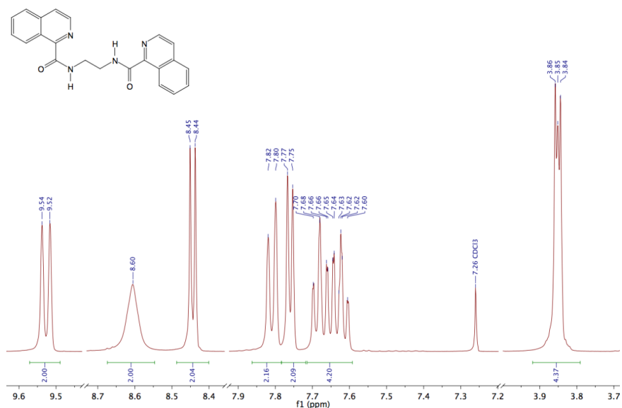
Figura 91. ^1\text{H} -RMN de Bis(1-isoquinolicarboxamido)etano ( 1a ).
