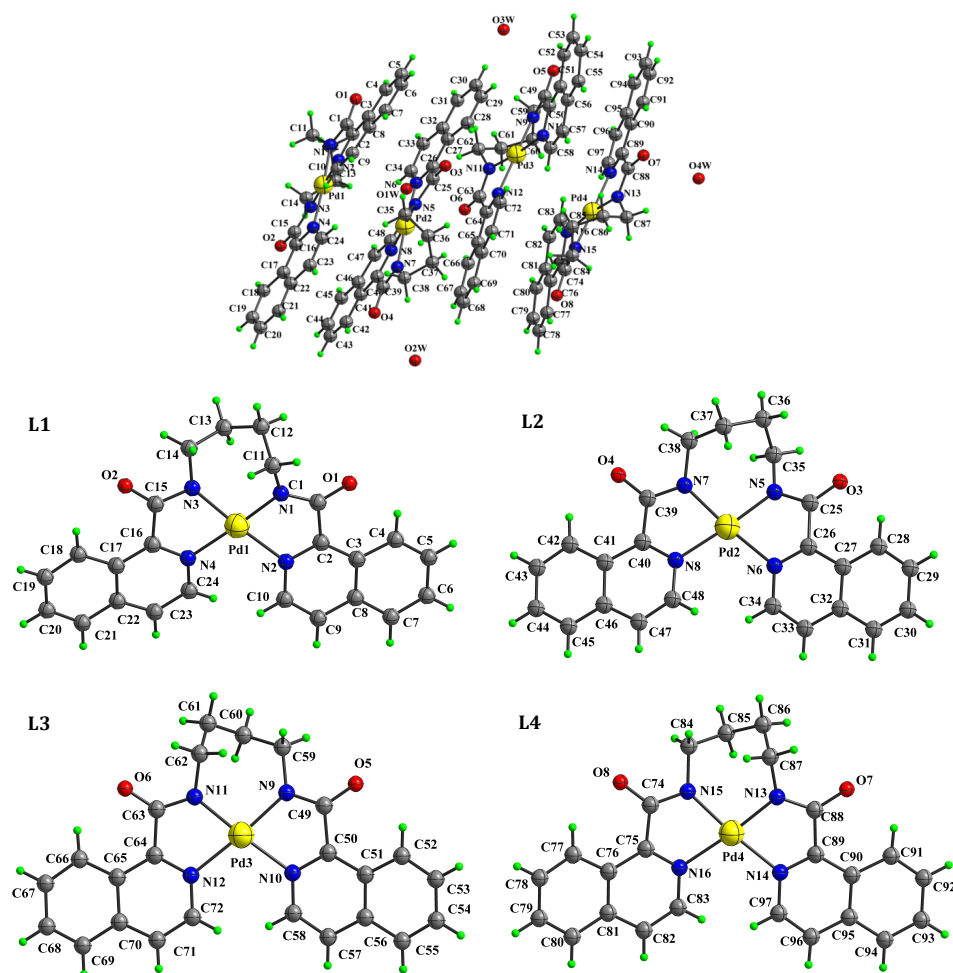
Figura 65. Unidad asimétrica de 7c . Se representa a cada cadena de forma individual para mayor claridad.
