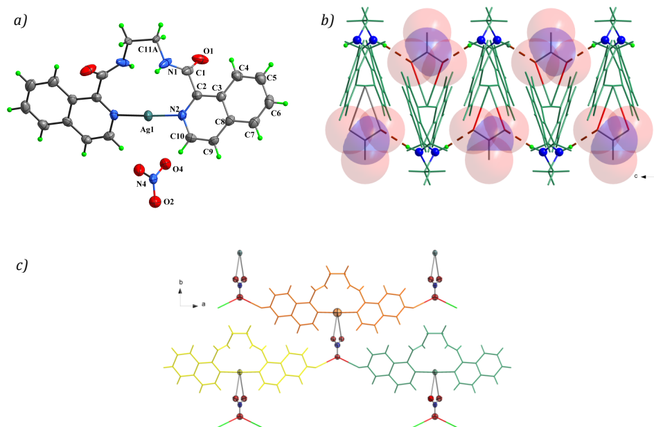
Figura 41. Representación estructural de 5a , a) Unidad asimétrica b) Conexión de la red 2D en el eje c vía \text{N-H}\cdots\text{O}_{(\text{nitrato})} c) Red 2D vía \text{C-H}\cdots\text{O}_{(\text{nitrato})} en el plano ab , cada cadena se representa de un color diferente para mayor claridad.
