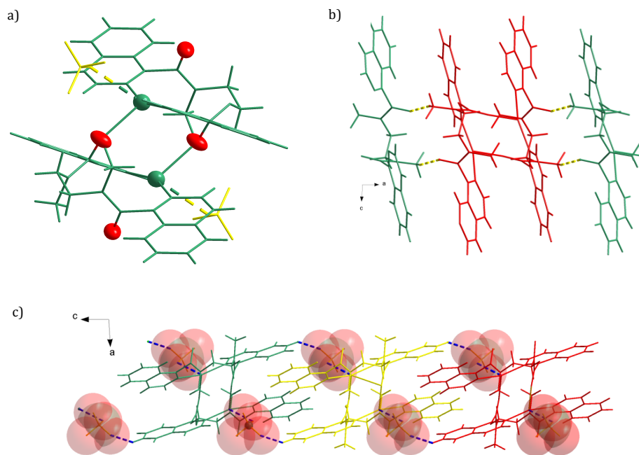
Figura 52. Empaquetamiento cristalino de 4g . a) Unidad dinuclear generada entre uniones coordinativas Ag(1)-O (amida) . b) Conexión de unidades dinucleares por medio de interacciones Csp 3 H...O (amida) a lo largo del eje a . c) Conexión de unidades dinucleares por medio de interacciones Ag-O (perclorato) y CH...O (perclorato) a lo largo del eje c .
