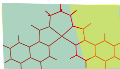
Figura 88. Compuesto 7b . Ángulo diedro generado entre los planos medios de los anillos de isoquinolina
