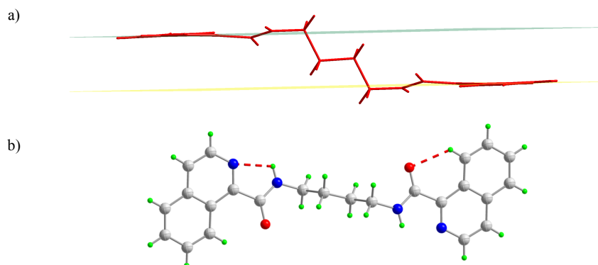
Figura 70. Compuesto 1c . a) Ángulo diedro generado entre los planos medios de los anillos de isoquinolina. b) Representación del enlace de hidrógeno intramolecular N-H (amida) ⋯N (isoquinolina)
