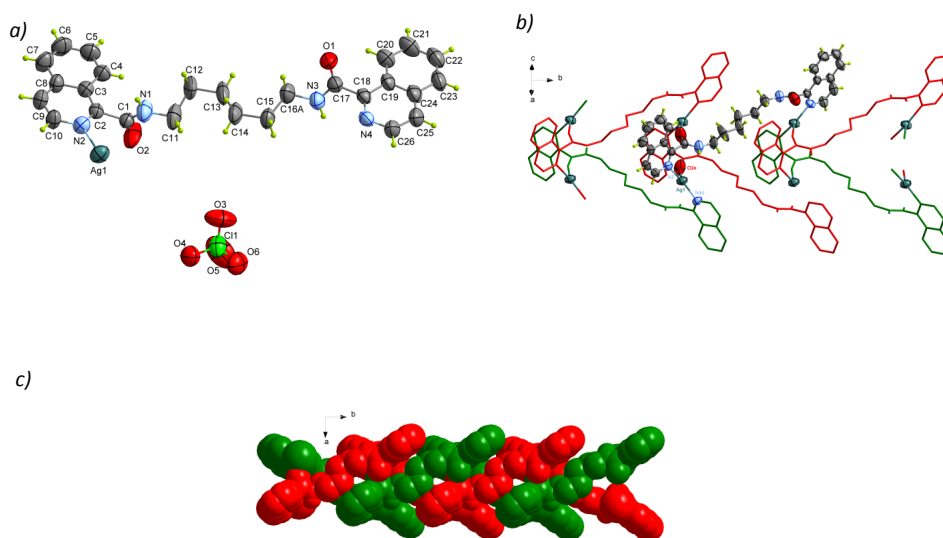
Figura 39. Representación estructural de 4e , a) Unidad asimétrica b) Cadena polimérica 1D, cada 1e se conecta a tres iones Ag(I) c) Vista en el eje b de la cadena polimérica. Notar que cada cadena polimérica, es una doble cadena y se forma por la unión en forma de un cierre con otra (rojo y verde).
