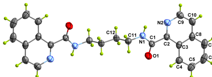
Figura 26. Representación molecular de 1c .
