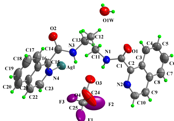
Figura 47. Unidad asimétrica del compuesto 6b .
