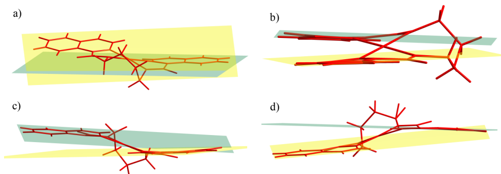
Figura 89. Compuesto 7b . Ángulo diedro generado entre los planos medios de los anillos de isoquinolina para cada uno de los ligandos de la unidad asimétrica a) L1 b) L2 c) L3 d) L4
