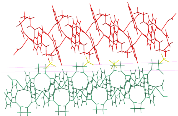
Figura 73. Compuesto 4a . a) Ángulo generado entre los planos medios de los anillos de isoquinolina. b) Distancia entre cadenas poliméricas 1D.
