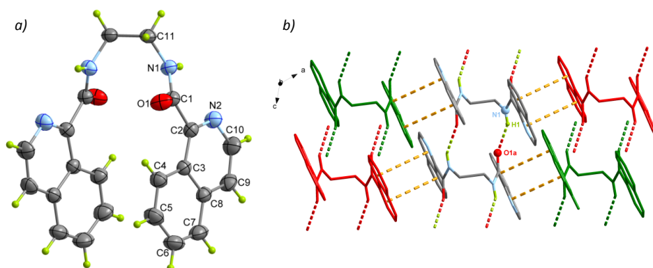
Figura 25. Representación molecular y estructural de 1a , a) Unidad asimétrica b) Interacción hojas \beta en el eje c y \pi-\pi en el plano ab .
