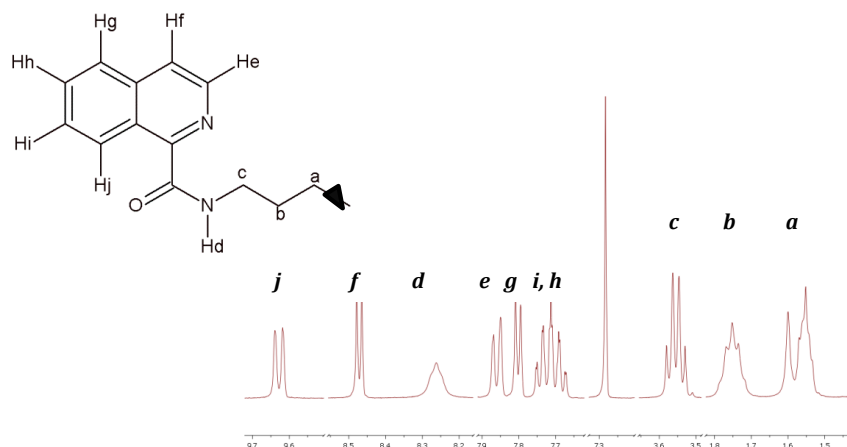
Figura 23. Espectros de ^1\text{H} -RMN (400 MHz, \delta ppm) de 1,6-bis(1-isoquinolincarboxamido)hexano ( 1e ).
