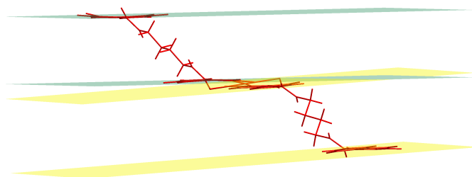
Figura 75. Compuesto 4c . Ángulo diedro generado entre los planos medios de los anillos de isoquinolina en colores diferentes para representar los dos ligandos en la unidad asimétrica del sistema.
