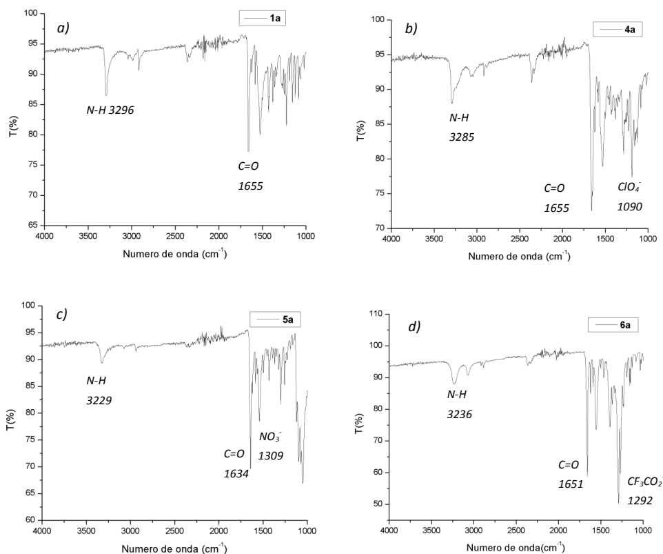
Figura 35. Espectro de infrarrojo de a) 1a donde se muestran las frecuencias de vibración de los grupos funcionales \text{NH}_{(\text{amida})} y \text{C}=\text{O}_{(\text{amida})} b), c) y d) se muestran además las tensiones correspondientes al contraión \text{ClO}_4^- , \text{NO}_3^- y \text{CF}_3\text{CO}_2^- respectivamente.
