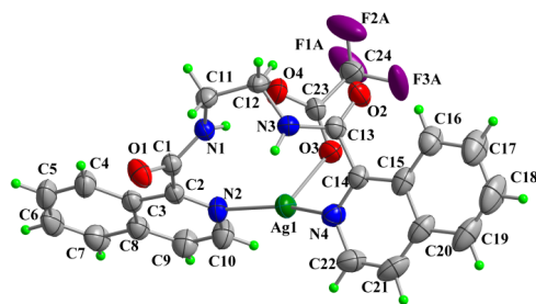
Figura 45. Unidad asimétrica del compuesto 6a .
