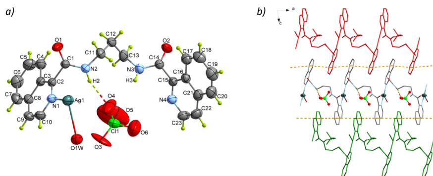
Figura 37. Representación estructural de 4b , a) Unidad asimétrica b) Cadenas poliméricas que se proyectan a lo largo del eje a y se conecta con otras cadenas por medio del apilamiento \pi - \pi .
