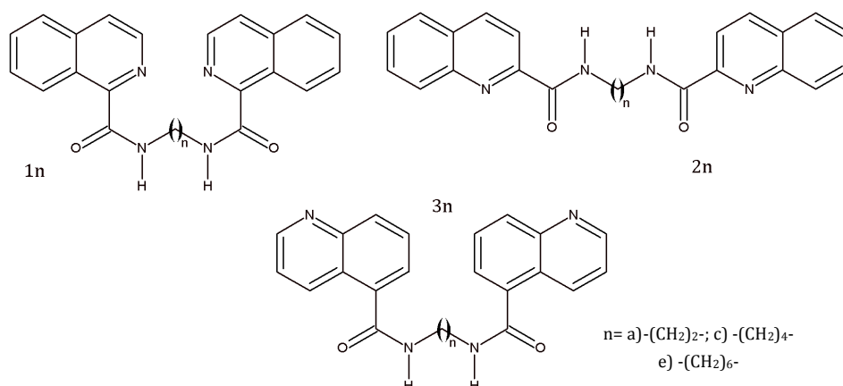
Figura 32. Representación estructural de las series 1n , 2n y 3n Mejorar
