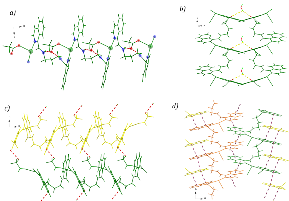
Figura 48. Empaquetamiento cristalino de 6b , a) Cadena Polimérica proyectada a lo largo del eje b , se incluye la interacción N-H\cdots O_{(\text{contraion})} como líneas punteadas en rojo b) Interacción O_{(\text{amida})}\cdots O_{(\text{agua})}\cdots O_{(\text{amida})} proyectada en el eje de polimerización c) Conexión de cadenas poliméricas por medio de interacciones de enlace halógeno C-H\cdots F a lo largo del eje c d) Interacción \pi-\pi que conecta cadenas en el plano ab .
