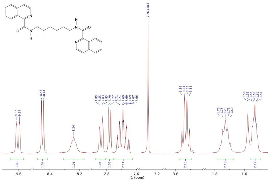
Figura 95. ^1\text{H} -RMN de Bis(1-isoquinolicarboxamido)etano ( 1e ).
