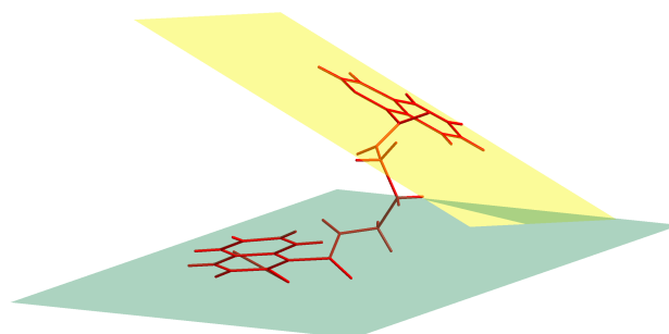
Figura 74. Compuesto 4b . Ángulo diedro generado entre los planos medios de los anillos de isoquinolina.
