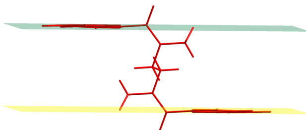
Figura 83. Compuesto 1g . Ángulo diedro generado entre los planos medios de los anillos de isoquinolina
