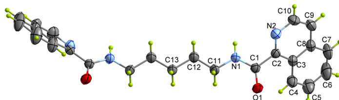
Figura 30. Representación molecular del ligando orgánico 1d .
