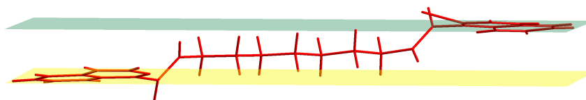
Figura 77. Compuesto 4f . Ángulo diedro generado entre los planos medios de los anillos de isoquinolina.
