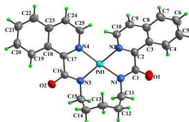
Figura 67. Unidad asimétrica del compuesto 7d .
