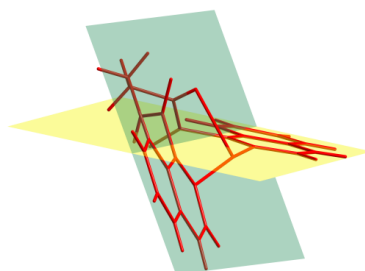
Figura 81. Compuesto 6a . Ángulo diedro generado entre los planos medios de los anillos de isoquinolina.
