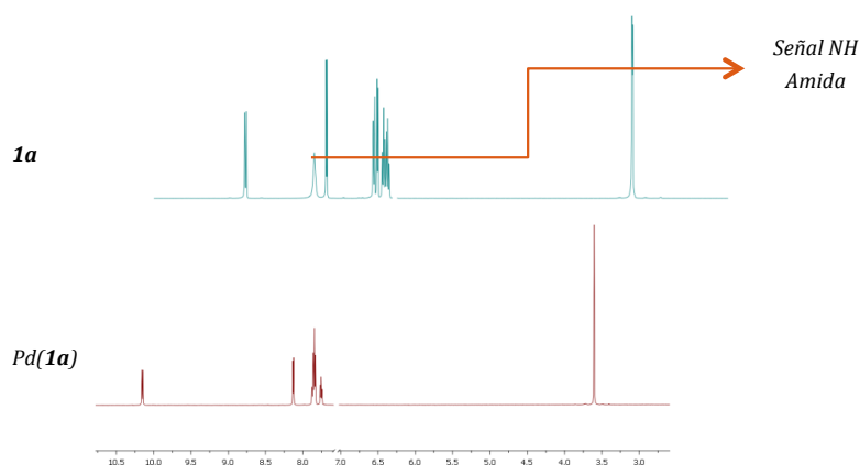
Figura 60. Superposición de los espectros de 1 H-RMN en CDCl 3 de los compuestos 1a y 7a .
