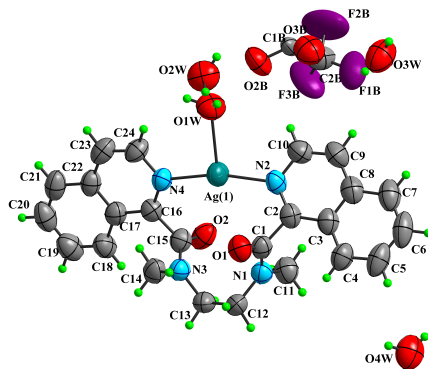
Figura 55. Unidad asimétrica del compuesto 6g .
