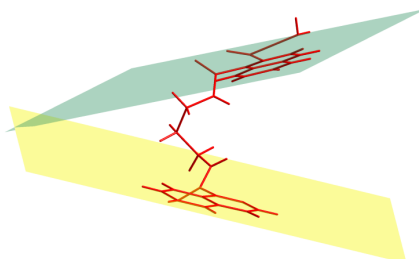
Figura 82. Compuesto 6b . Ángulo diedro generado entre los planos medios de los anillos de isoquinolina
