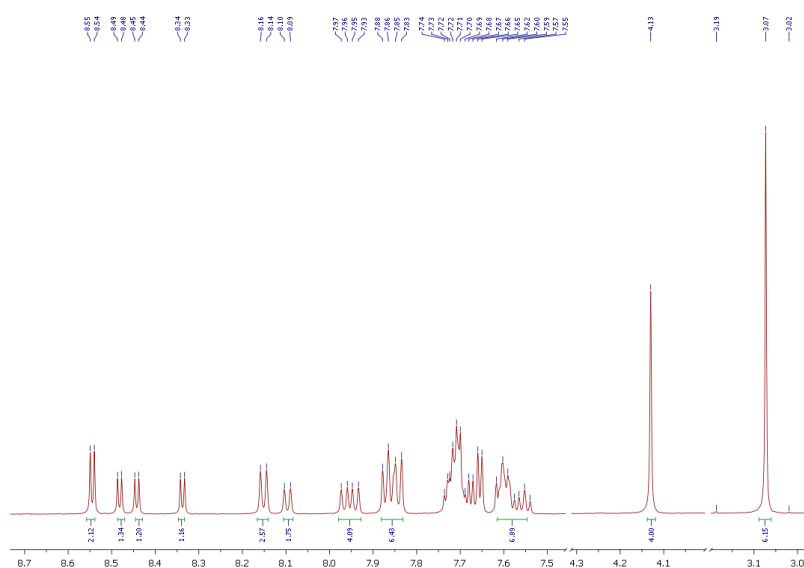
Figura 97. ^1\text{H} -RMN de N, N' -dimetil-Bis(1-isoquinolicarboxamido)etano ( 1g ).
