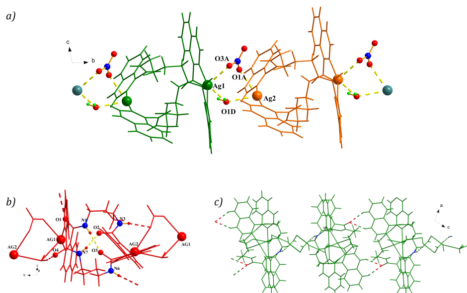
Figura 44. Empaquetamiento cristalino de 5c , a) Conexión entre dímeros a lo largo del eje b , b) Interacción de enlace de hidrógeno intramolecular amida-amida en color amarillo y en rojo la interacción entre el grupo amida y los iones nitrato y molécula de agua de solvatación c) Empaquetamiento por medio de CH \cdots O (amida) y NH \cdots O (nitrato) en el plano ac .
