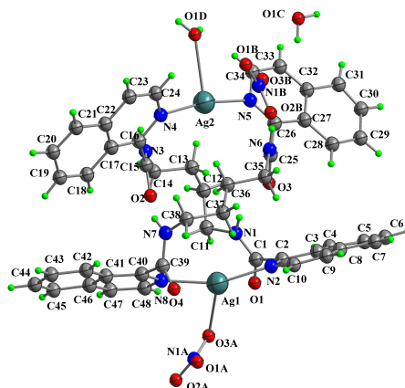
Figura 43. Unidad asimétrica del compuesto de coordinación 5c .
