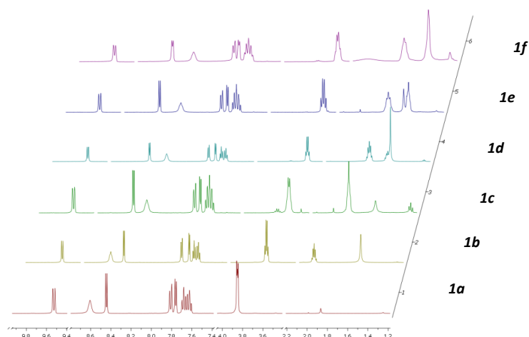
Figura 22. Espectros de ^1\text{H} -RMN (400 MHz, \delta ppm), de las bisamida secundarias.
