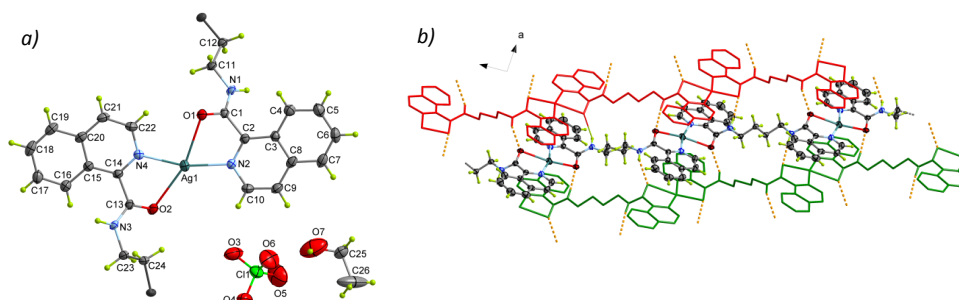
Figura 38. Representación estructural de 4c , a) Unidad asimétrica b) Cadena poliméricas que se conectan por medio de enlaces de hidrógeno definiendo un shintón en Hojas \beta .
