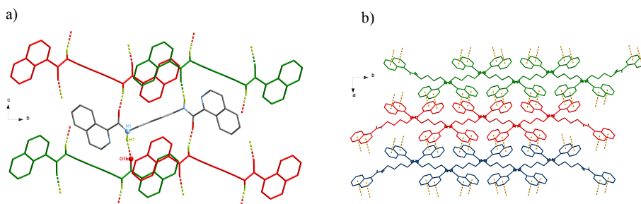
Figura 27. Empaquetamiento cristalino de 1c . a) Representación de la red 4,4 generada a partir de interacciones NH-O (amida) en el plano bc . b) Representación de tres capas generadas a través de redes 4,4 a lo largo del plano bc . Cada capa es conectada a otras dos capas por medio de interacciones \pi - \pi a lo largo del eje a .
