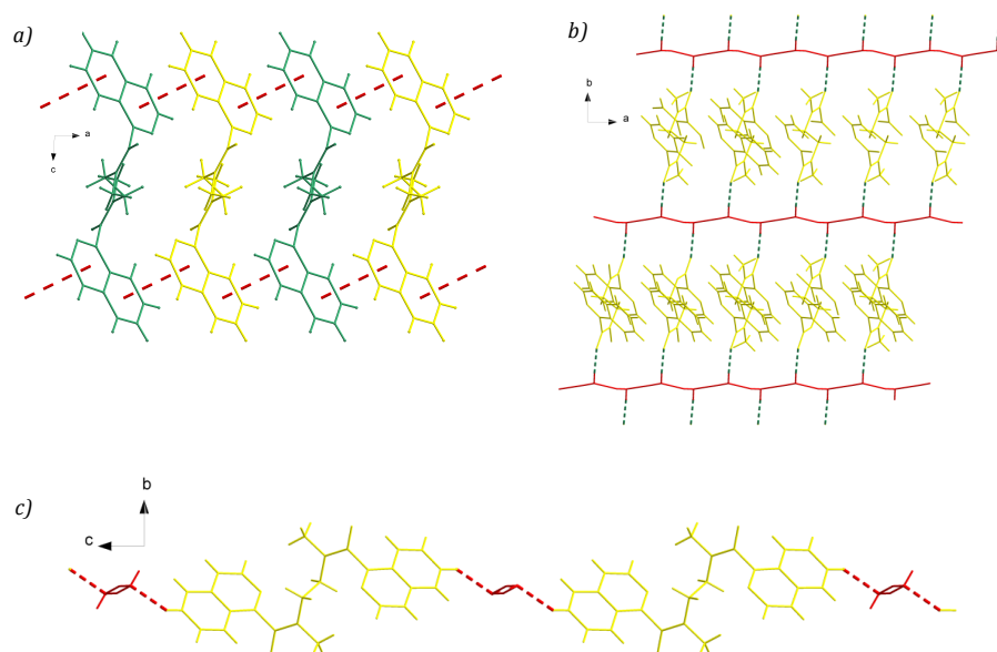
Figura 50. Empaquetamiento cristalino de 1g . a) Interacción \pi - \pi a lo largo del eje a . b) Conexión de cadenas generadas por apilamiento \pi - \pi a través de enlaces de hidrógeno entre oxígenos del grupo amida y las moléculas de agua de cristalización. b) Unión de 1g por medio de interacciones C-H \cdots O (agua) a lo largo del eje c .
