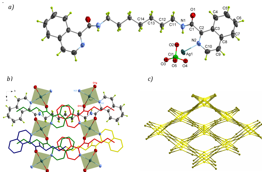
Figura 40. Representación estructural de 4f , a) Unidad asimétrica b) Empaquetamiento cristalino 3D del polímero de coordinación de Ag(I) c) Topología [4^2 8^4]\text{-pts} , donde cada ion metálico actúa como un nodo de cuatro ejes y el ligando como un conector de cuatro ejes.
