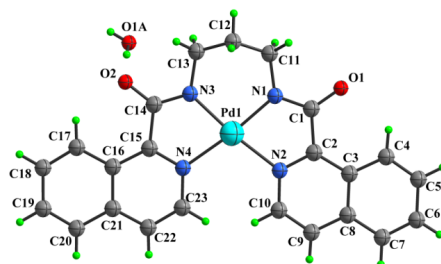
Figura 63. Unidad asimétrica del compuesto 7b .
