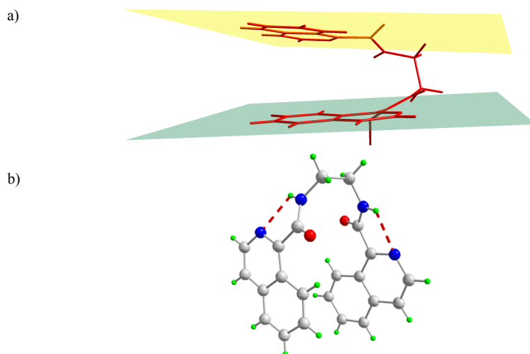
Figura 69: Compuesto 1a . a) Ángulo diedro generado entre los planos medios de los anillos de isoquinolina. b) Representación del enlace de hidrógeno intramolecular N-H (amida) ⋯N (isoquinolina)
