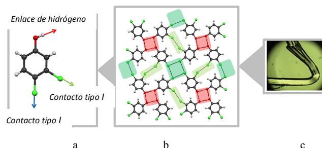
Figura 7. La estructura cristalina del 3,4-diclorofenol es sustentada por (a) el sintón primario de enlace de hidrógeno (rojo) y dos contactos tipo I y II. (b) El aislamiento del enlace de hidrógeno del halógeno resulta en (c) la propiedad plástica del compuesto sin la fractura del material. 14
