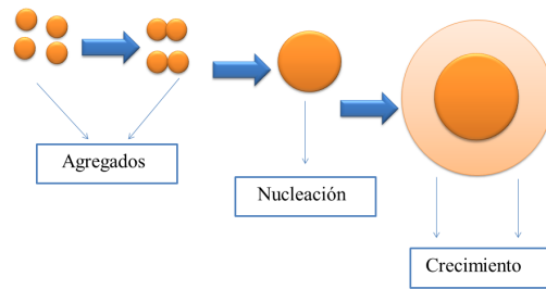
Figura 3. Proceso de Cristalización paso a paso en solución.
