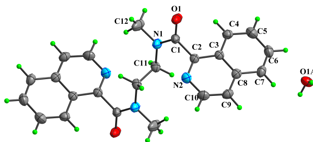
Figura 49. Unidad asimétrica del compuesto 1g .
