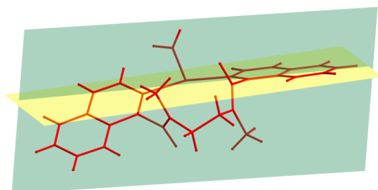
Figura 86. Compuesto 6g . Ángulo diedro generado entre los planos medios de los anillos de isoquinolina.
