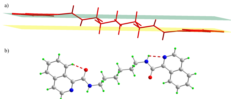
Figura 72. Compuesto 1e . a) Ángulo diedro generado entre los planos medios de los anillos de isoquinolina. b) Representación del enlace de hidrógeno intramolecular N-H (amida) ···N (isoquinolina) .
