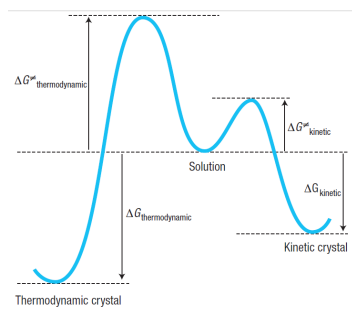
Figura 4. Principio de Curtin-Hammontt. Existen dos posibles caminos para una reacción, el cinético, en donde la reacción es rápida debido a la baja energía de activación que resulta en estructuras que no son de mínima energía y el termodinámico proceso más lento debido a la elevada energía de activación que produce una estructura de mínimo de energía. 15
