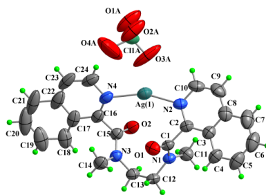
Figura 51. Unidad asimétrica del compuesto 4g .
