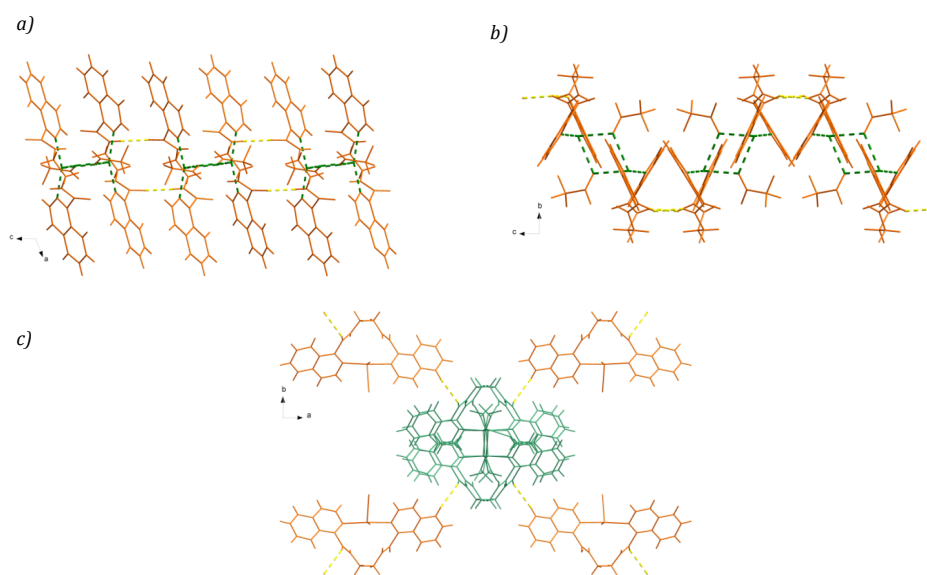
Figura 46. Empaquetamiento cristalino de 6a , a) y b) Conexión de monómeros a lo largo del eje c por medio de interacciones Ag-O-Ag en color verde y N-H \cdots O en amarillo c) Conexión de las hojas b de unidades mononucleares por medio de la interacción CH \cdots O (amida) color amarillo.
