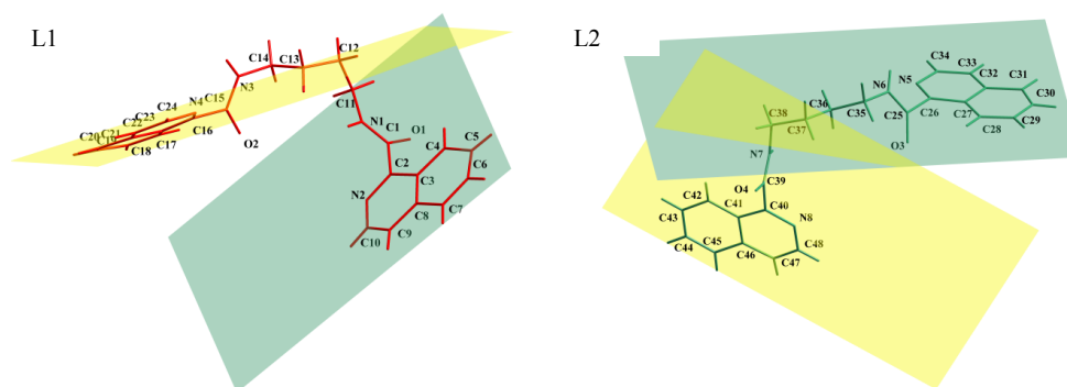
Figura 80. Compuesto 5c . Ángulo diedro generado entre los planos medios de los anillos de isoquinolina, se representan los dos ligandos L1 y L2 de la unidad asimétrica por separado por mayor claridad.
