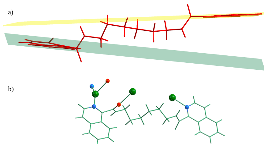
Figura 76. Compuesto 4e . a) Ángulo diedro generado entre los planos medios de los anillos de isoquinolina. b) Representación del ligando 4e coordinando a tres centros metálicos de plata(I).
