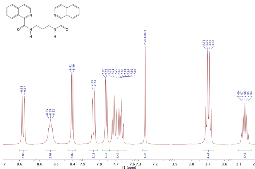
Figura 92. ^1\text{H} -RMN de Bis(1-isoquinolicarboxamido)etano ( 1b ).
