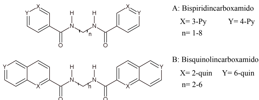
Figura 12. Representación de Bispiridilcarboxamido y Bisquinolincarboxamido
