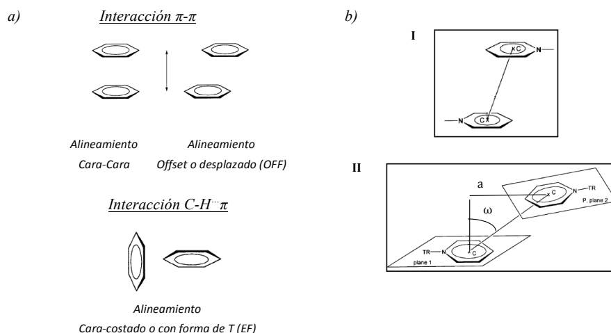
Figura 8. (a) Principales orientaciones de las interacciones aromáticas. 1 (b) Parámetros de interacción aromática en sistemas piridinicos I) Distancia centroide-centroide Cg \cdots Cg con valores típicos entre 3.4 a 4.6 Å, II) ángulo de desplazamiento \omega (slip/ ^\circ ) cuyos valores preferenciales de 0 a 40 ^\circ y la distancia de desplazamiento a (slip/Å) con valores entre 0 y 4Å.
