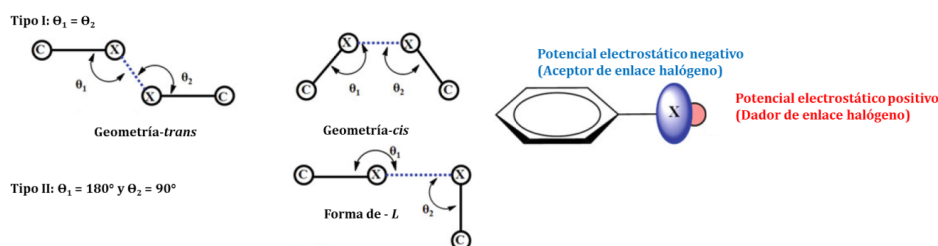
Figura 10. Representación geométrica del enlace halógeno. 37
