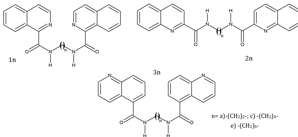
Figura 18. Representación estructural de las series 1n , 2n y 3n .
