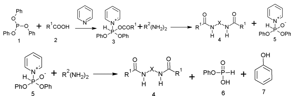
Figura 19. Mecanismo de reacción para la obtención de los compuestos del tipo bis(1-isoquinolincarboxamido)alcano.
