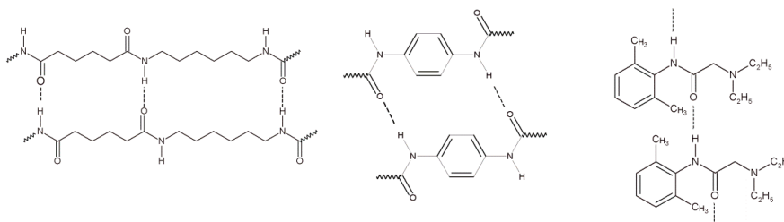
Figura 11. Representación de izquierda a derecha Nylon 6,6; Kevlar®; Lidocaína
