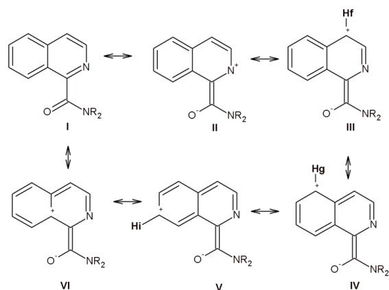
Figura 24. Deslocalización electrónica del grupo amida en el anillo isoquinolínico para los compuestos del tipo bis(1-isoquinolincarboxamido)alcano.
