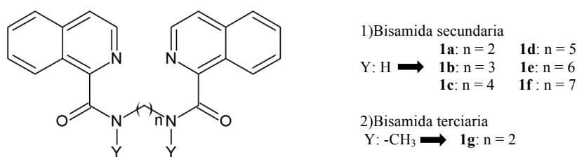
Figura 17. Serie homóloga de bisamidas del tipo bis(1-isoquinolincarboxamido)alcano.
