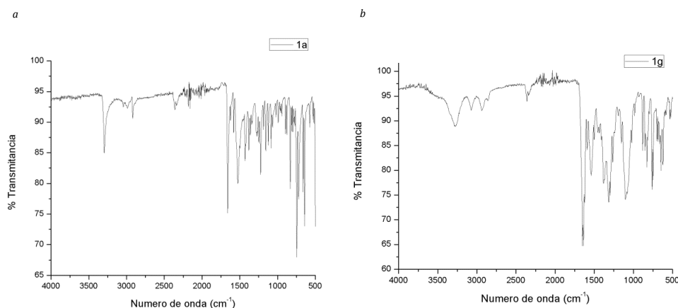
Figura 21. a) Espectro de Infrarrojo de los compuestos 1a y b) 1g .
