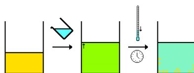
Figura 15. Representación ilustrativa de la cristalización por evaporación lenta.
