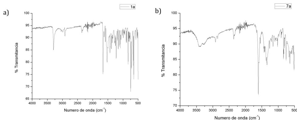
Figura 59. Espectros de infrarrojo de a) 1,2-bis(1-isoquinolinecarboxamido)etano ( 1a ) y [Pd( 1a )]·nH 2 O ( 7a ).
