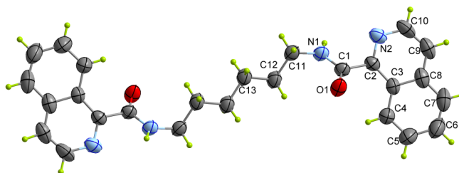
Figura 28. Representación molecular del ligando orgánico 1e
