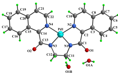
Figura 61. Unidad asimétrica del compuesto 7a .
