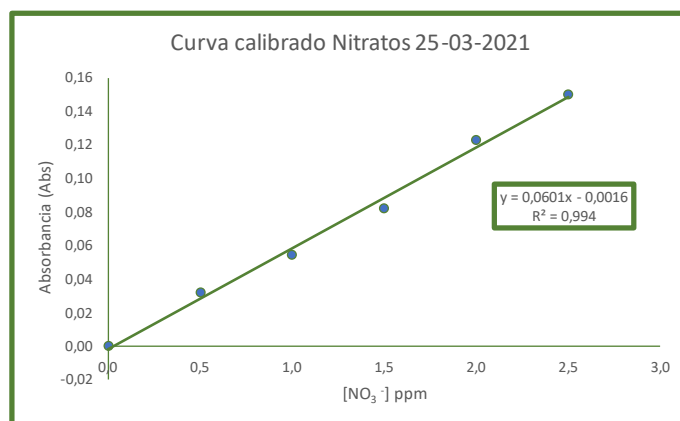
Figura 3. Curva de calibrado de nitratos en agua.
