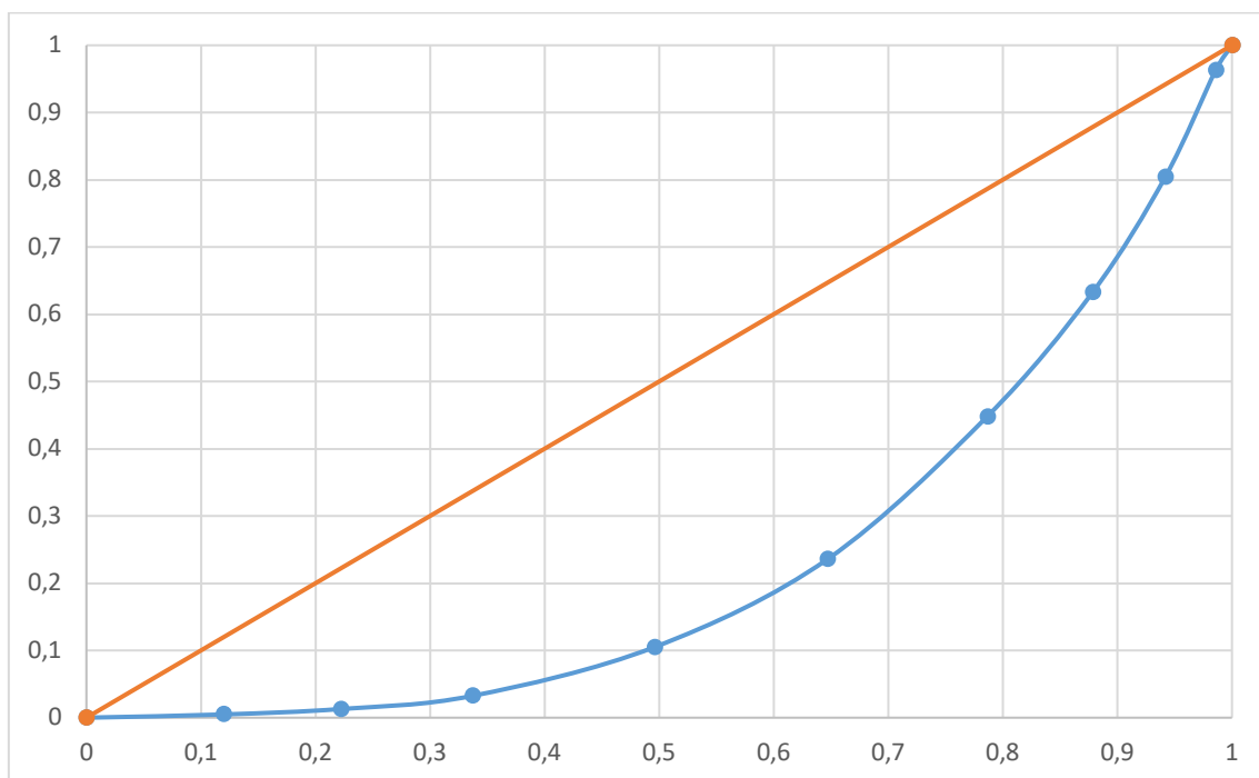
Curva Lorenz
