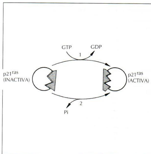
Fig. 2.—Ciclo de hidrólisis de GTP de la proteína p21 ras : la hidrólisis del GTP fijado a la proteína inactiva a ésta. La proteína GAP (que no aparece en la figura) promueve dicha hidrólisis, y por ello se dice que GAP es un regulador negativo de la actividad de p21 ras . El intercambio de GDP por GTP activa a p21 ras . La entrada de GTP está promovida por una proteína intercambiadora de nucleótidos de guanina (que tampoco aparece en la figura). Se han identificado proteínas homólogas a GAP y a la proteína intercambiadora de nucleótidos de guanina en diversos organismos ( levaduras , Drosophila melanogaster , Caenorhabditis elegans ), lo que indica que el mecanismo de activación-inactivación se ha conservado a lo largo de la evolución.
