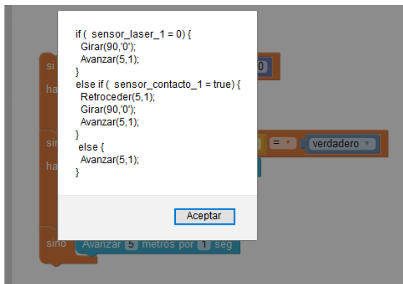
Figura 36: Ejemplo de funcionamiento del botón “Mostrar Código”
