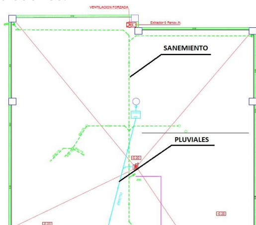
Figura 32: Instalación de saneamiento en planta garaje. Fuente: Proyecto original.
