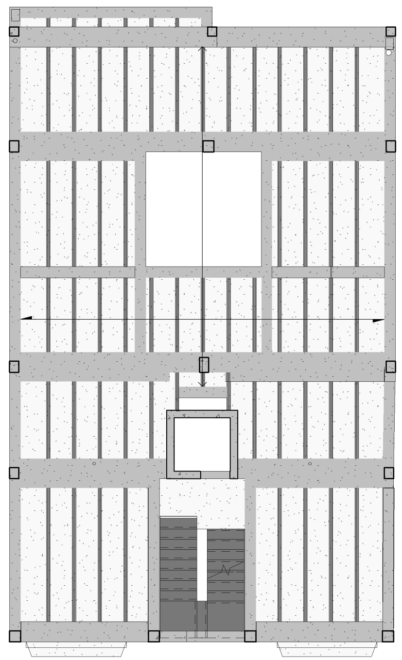
FORJADO 3 COTA DE ENCOFRADO: +8,35 m.
