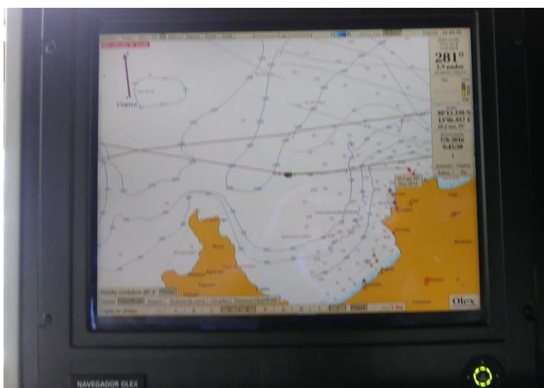
Fig. 40: Navegador OLEX. Fuente: Elaboración propia
