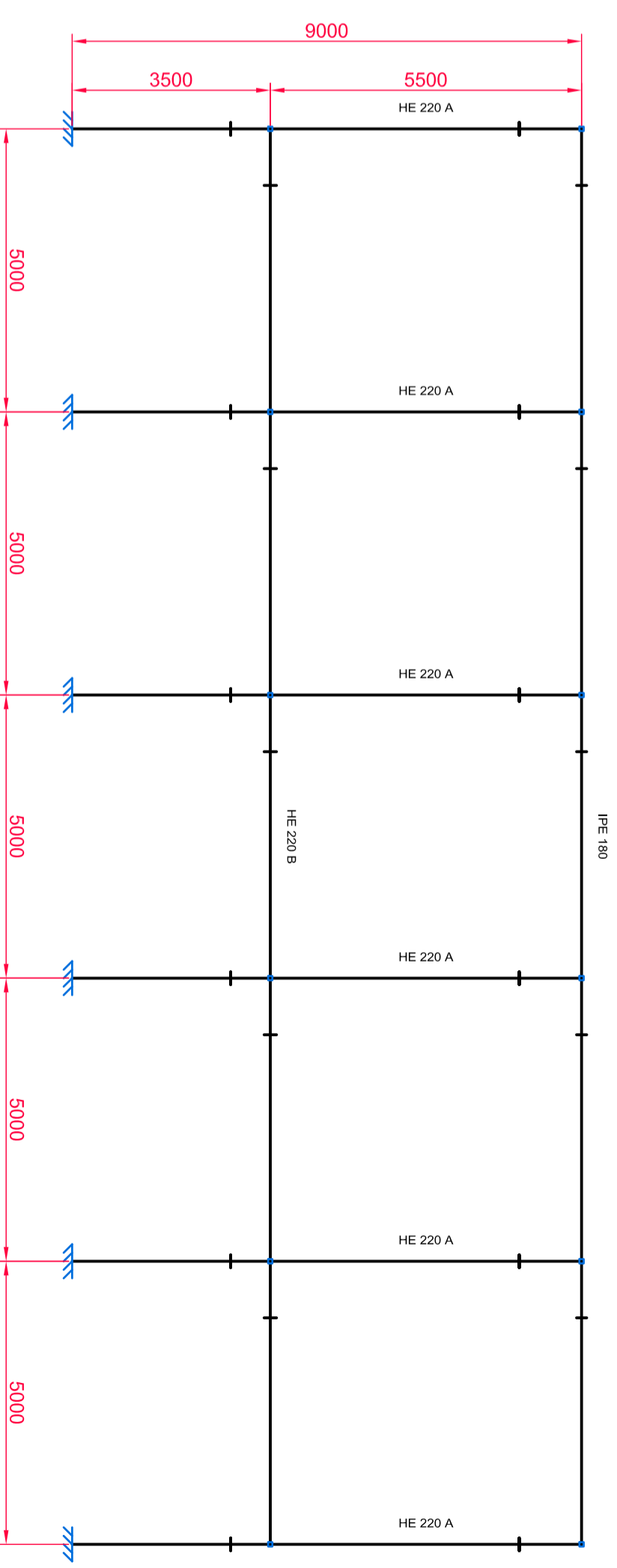
Pórtico P8
