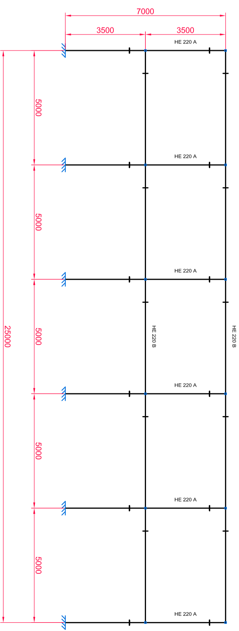
Pórtico P2
