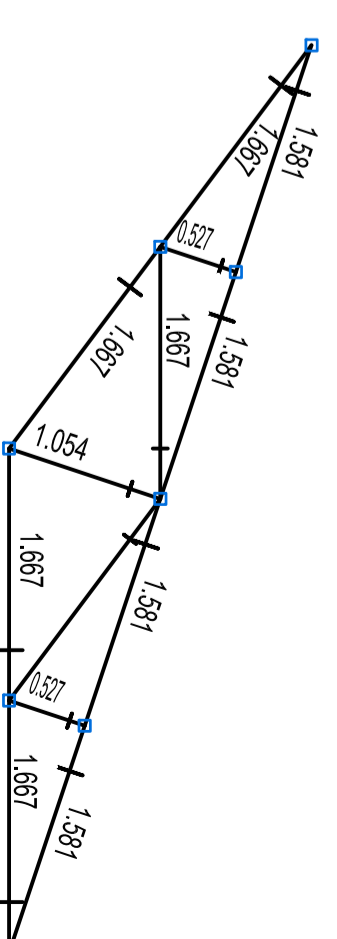
DETALLE LONGITUDES DE LAS BARRAS DE LA CELOSÍA
