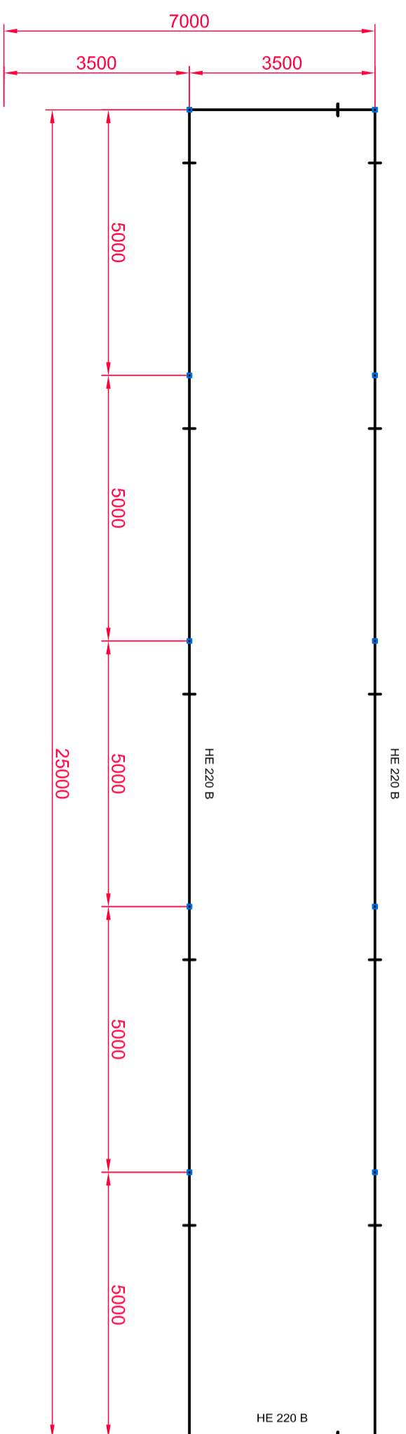
Pórtico P1 (Volado)
