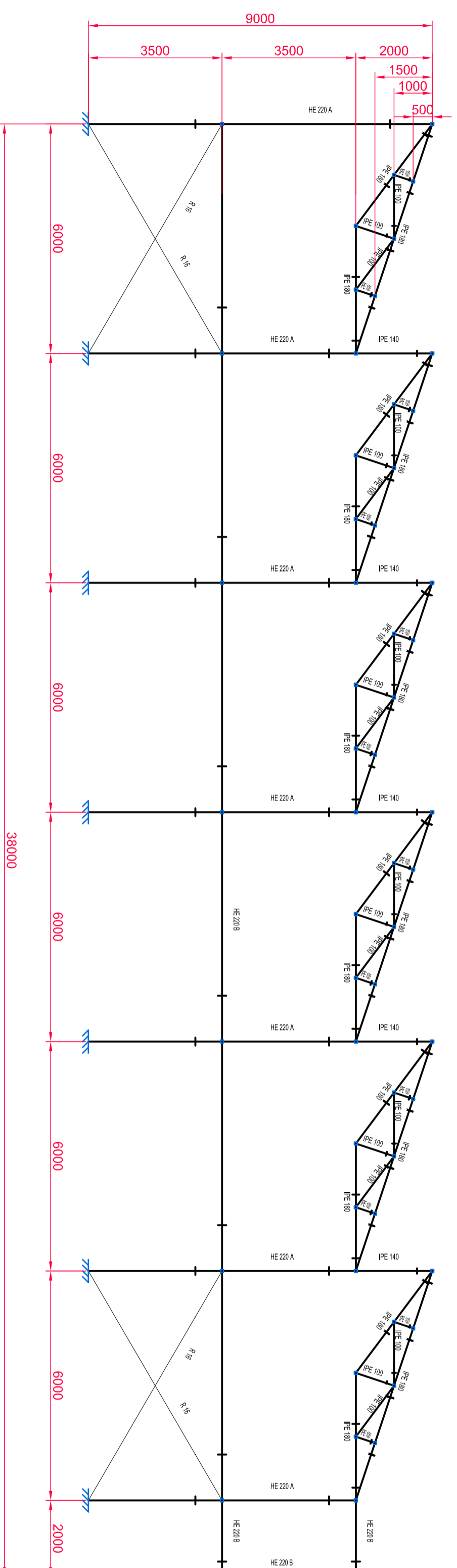
DETALLE LONGITUDES DE LAS BARRAS DE LA CELOSÍA
